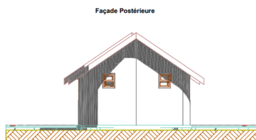
Façades des bungalows
